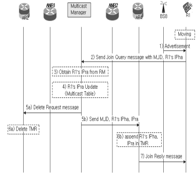
Fig. 10. Message Flow
