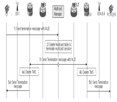
Fig. 12. Message Flow
